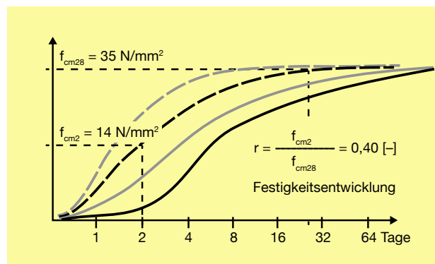
Bild 3: Festigkeitsentwicklung verschiedener Betone
