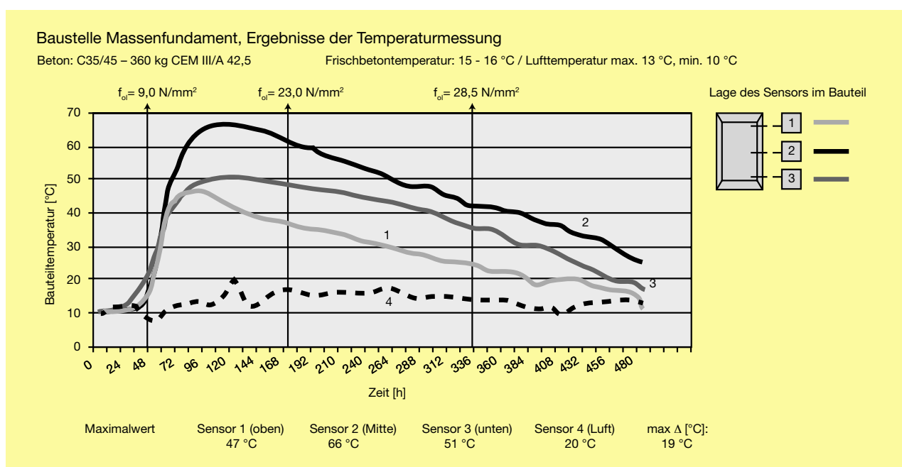
Bild 9: Beispiel für Temperaturmessungen im Bauteil
