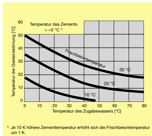
Bild 6: Grafische Abschätzung der zu erwartenden Frischbetontemperatur
