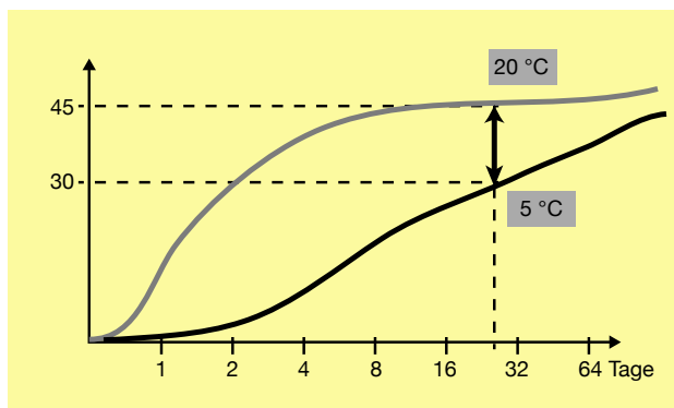
Bild 2: Verzügerte Druckfestigkeitsentwicklung eines Betons in Abhängigkeit der Temperatur (Beispiel)
